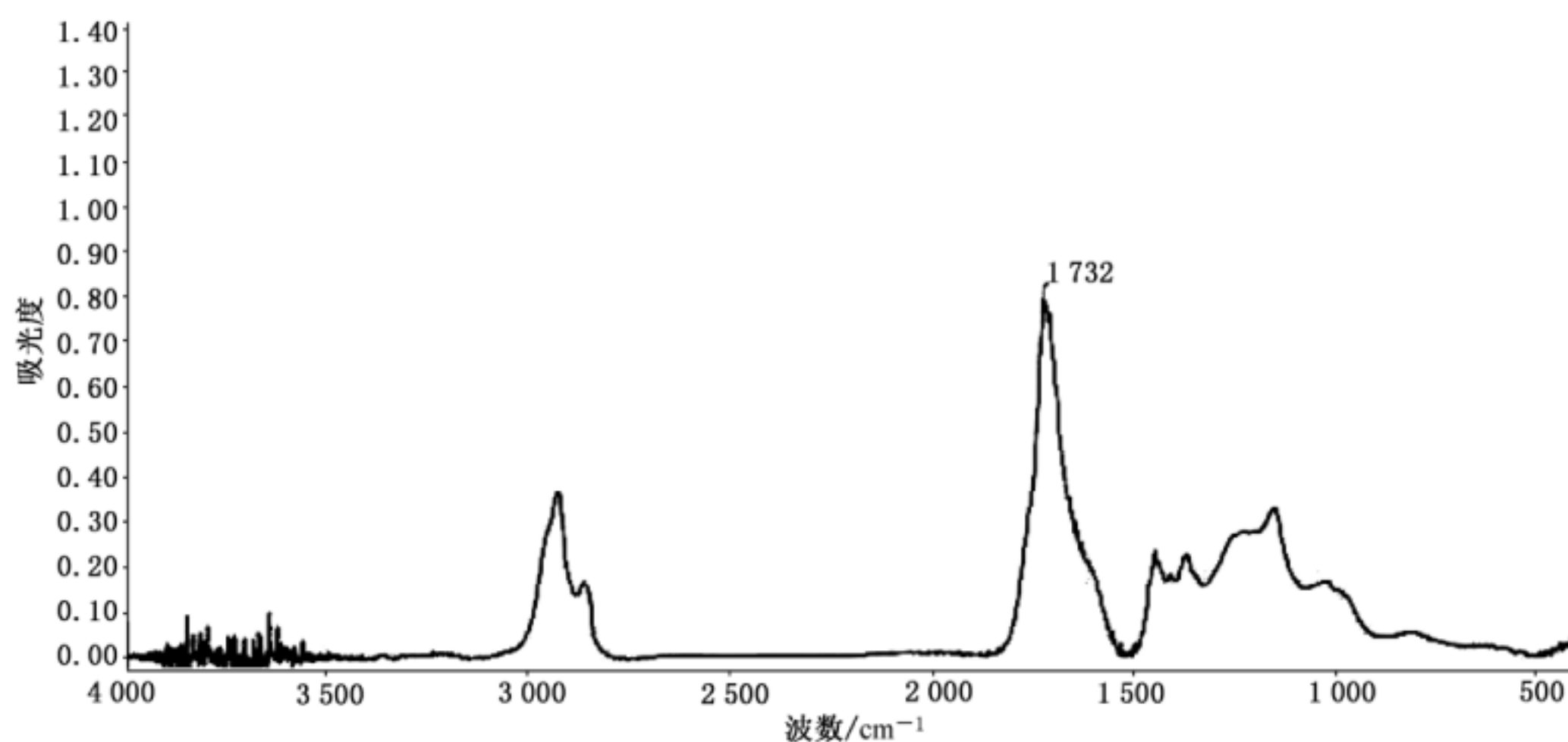
图 A.26 热处理改变颜色后波罗的海琥珀(红色)的特征红外光谱
