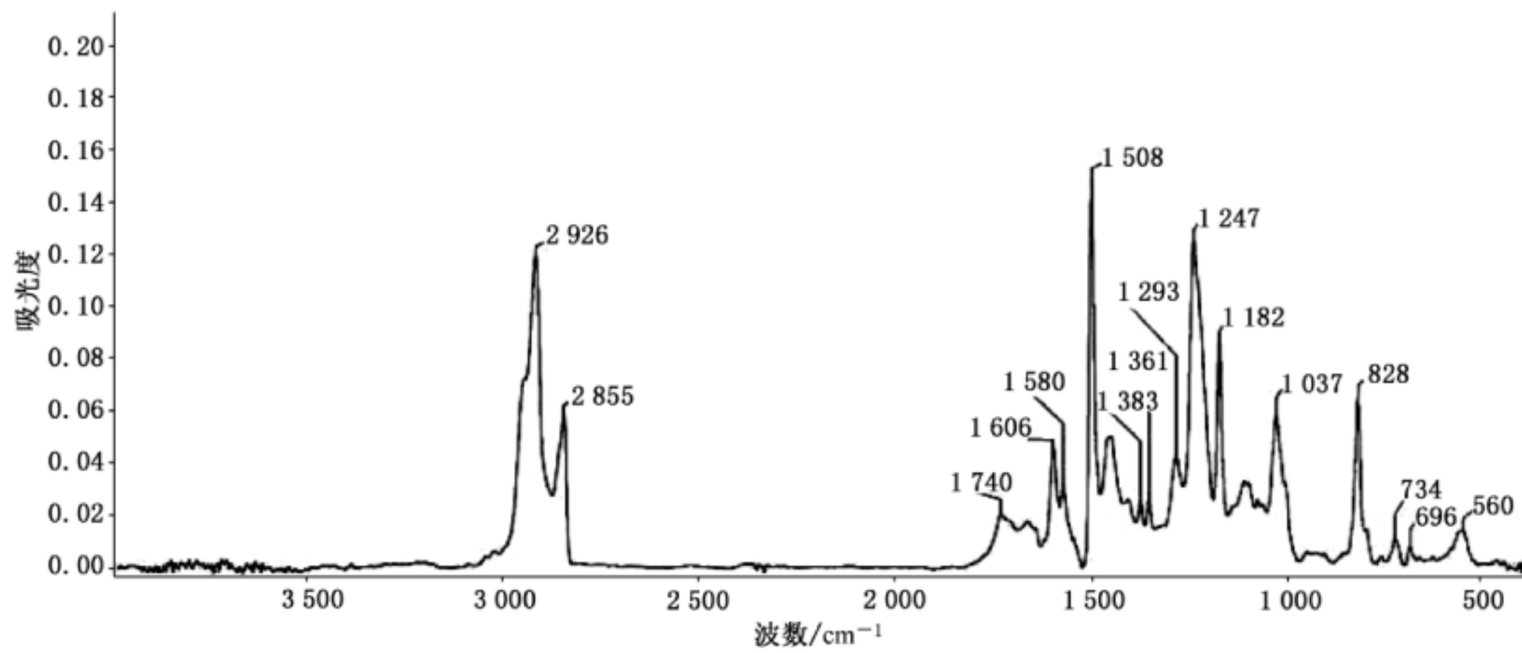
图 A.11 仿琥珀(环氧树脂类)的特征红外光谱
