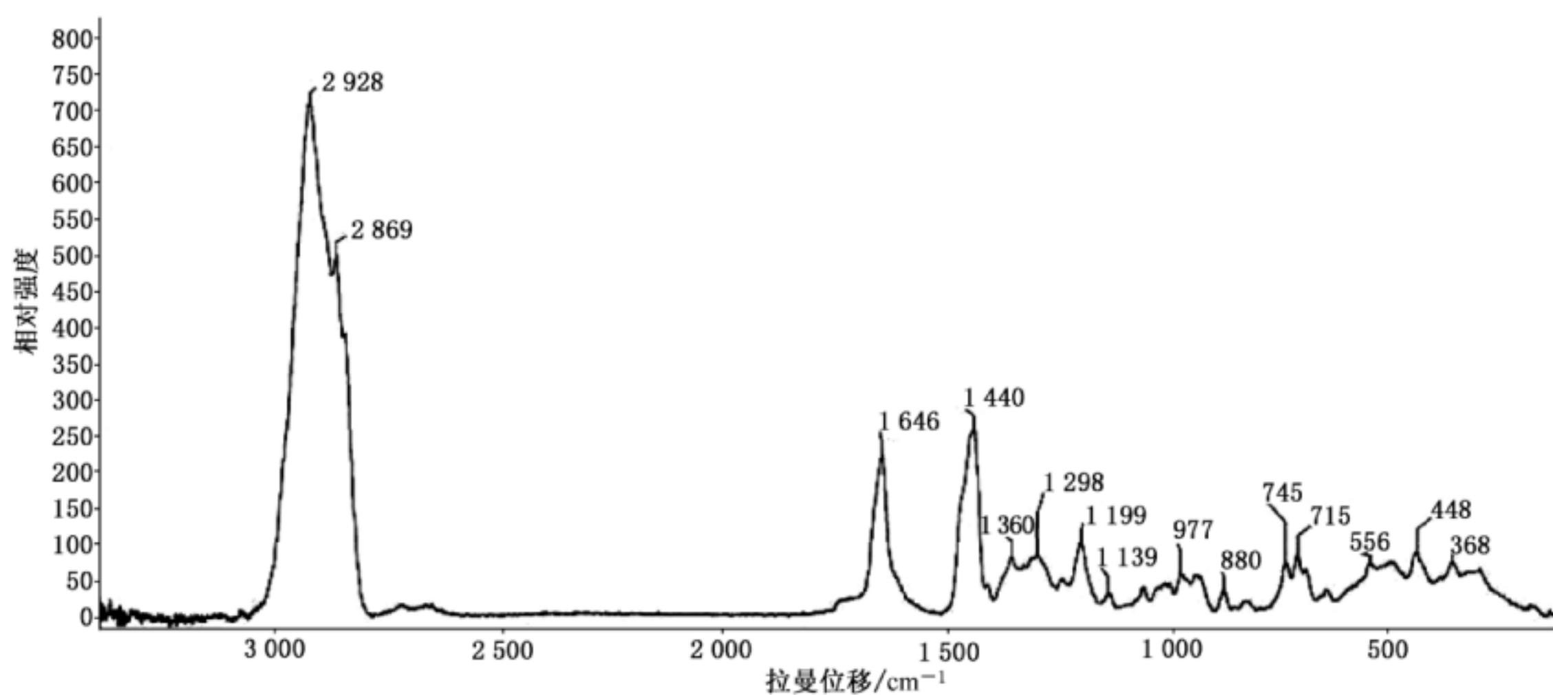
图 A.13 波罗的海琥珀的特征拉曼光谱
