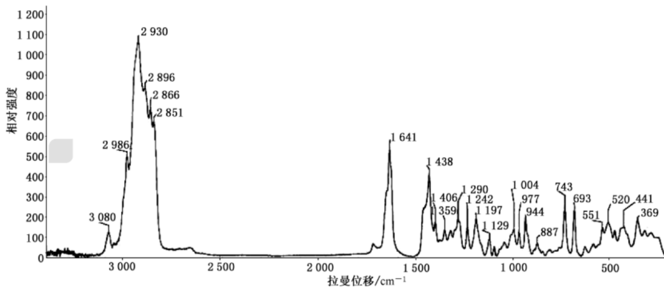
图 A.21 马达加斯加半石化树脂的特征拉曼光谱
