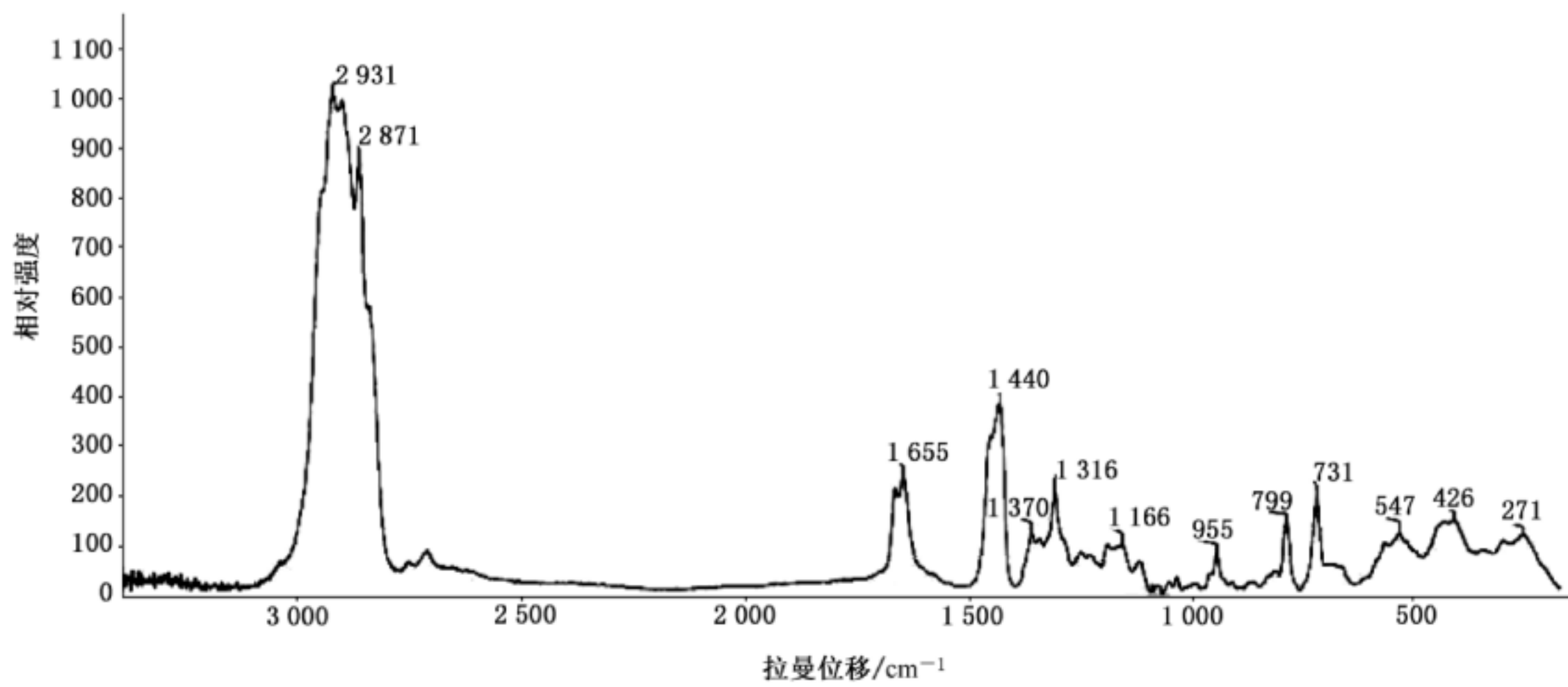
图 A.20 婆罗洲半石化树脂的特征拉曼光谱
