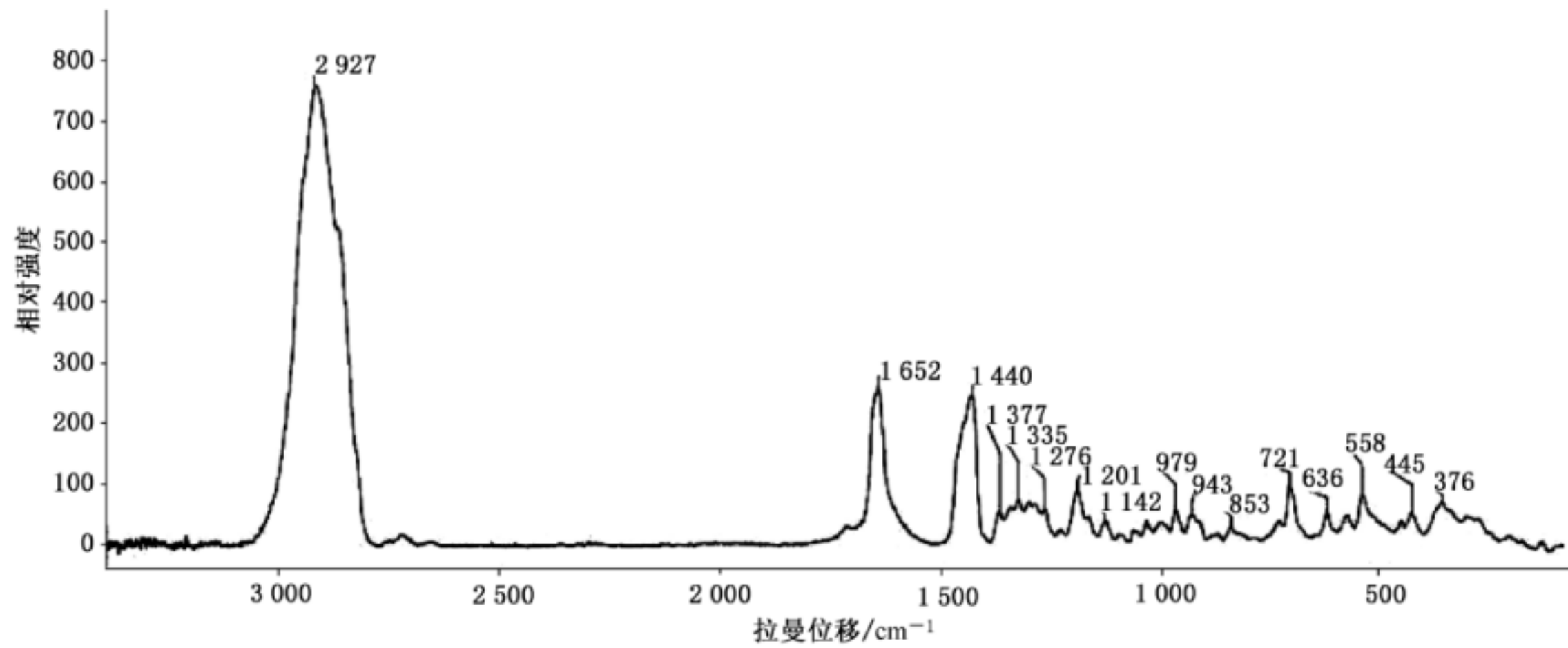
图 A.15 多米尼加琥珀的特征拉曼光谱
