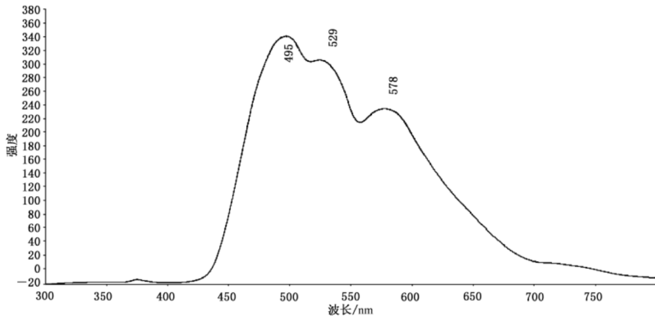
图 A.28 经辐照波罗的海琥珀(橙红色)的特征荧光光谱
