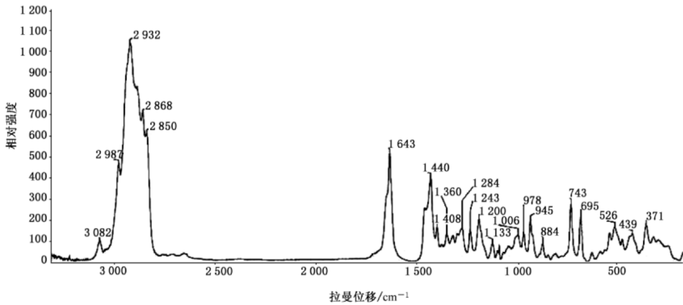
图 A.19 哥伦比亚半石化树脂的特征拉曼光谱
