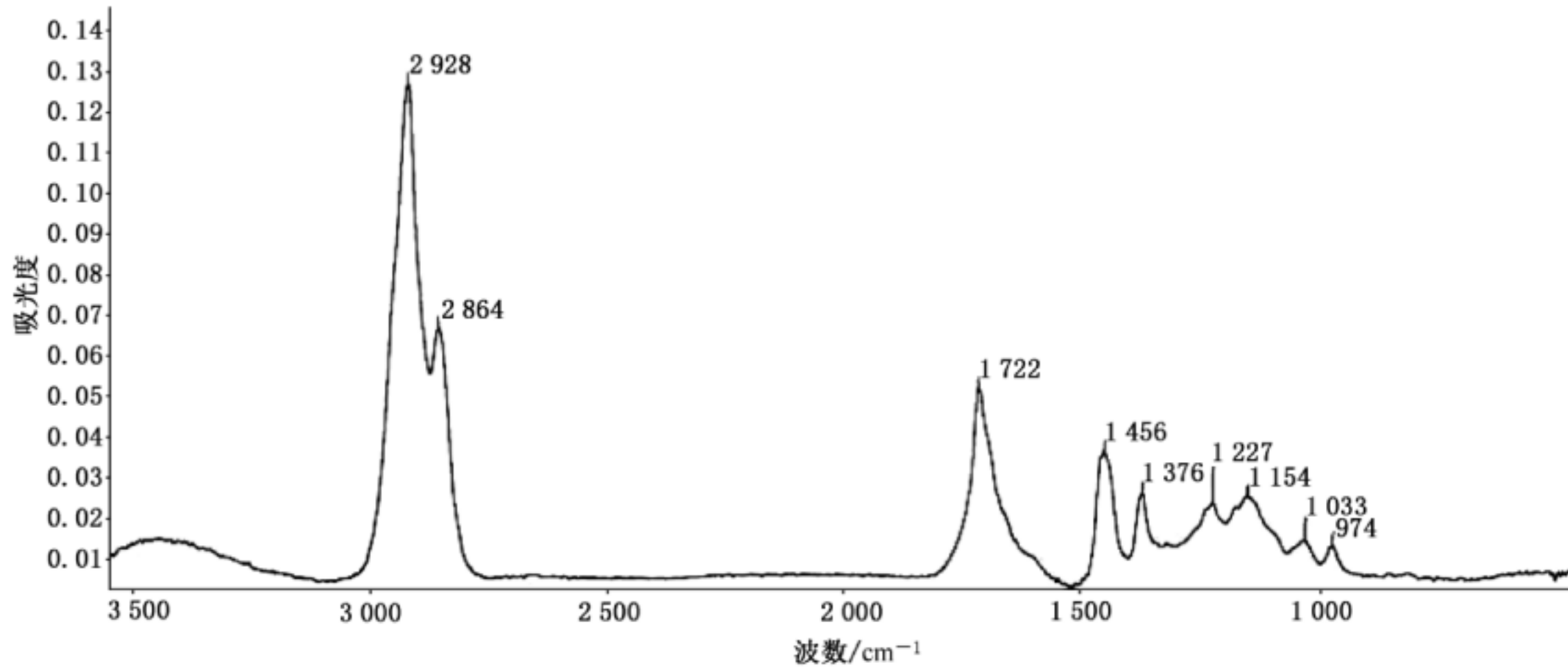
图 A.5 缅甸琥珀的特征红外光谱
