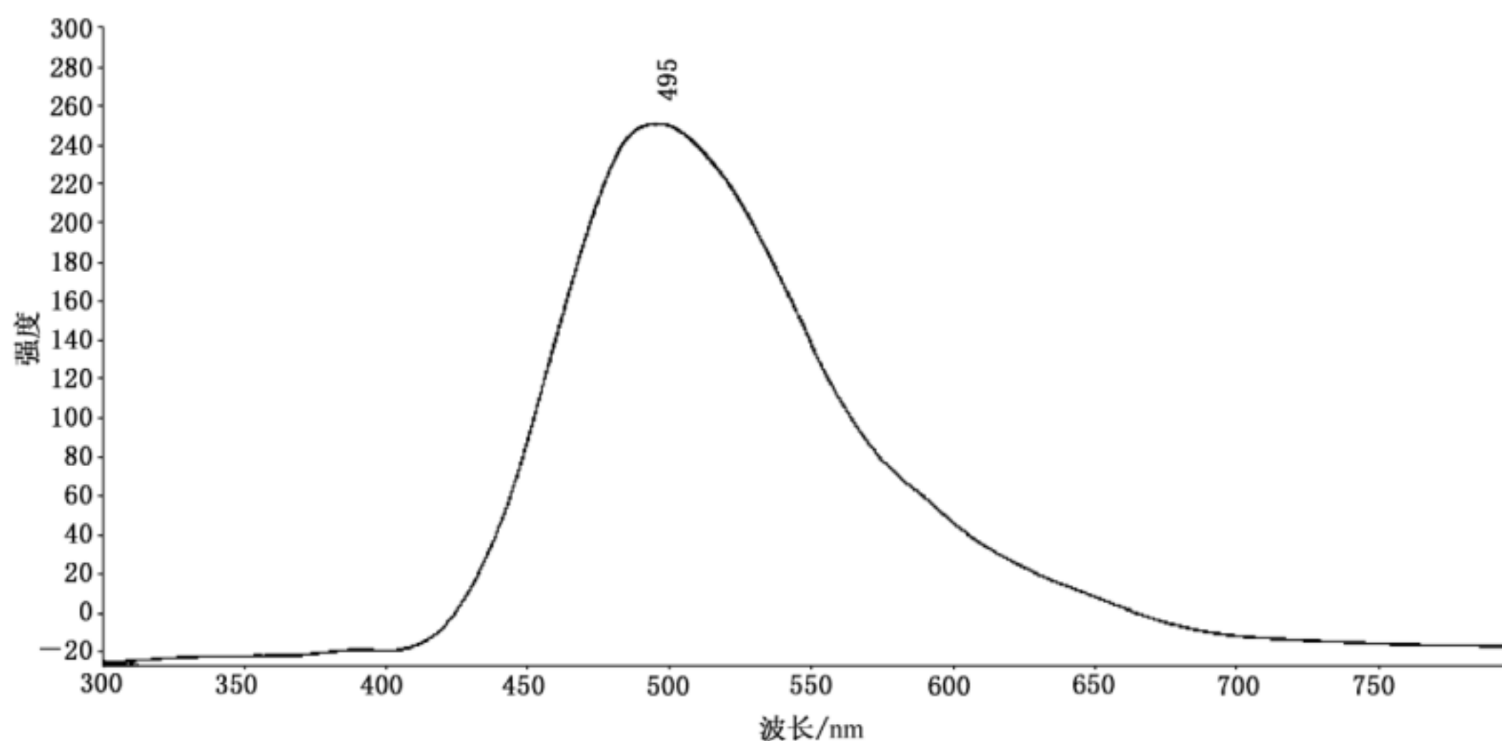
图 A.27 未经辐照波罗的海琥珀(黄色)的特征荧光光谱
