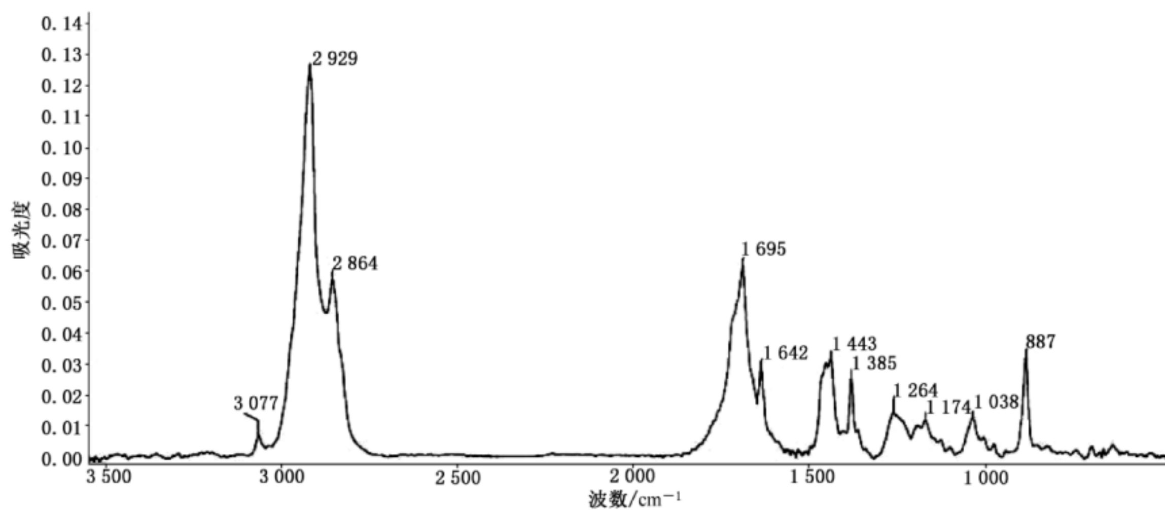
图 A.7 哥伦比亚半石化树脂的特征红外光谱
