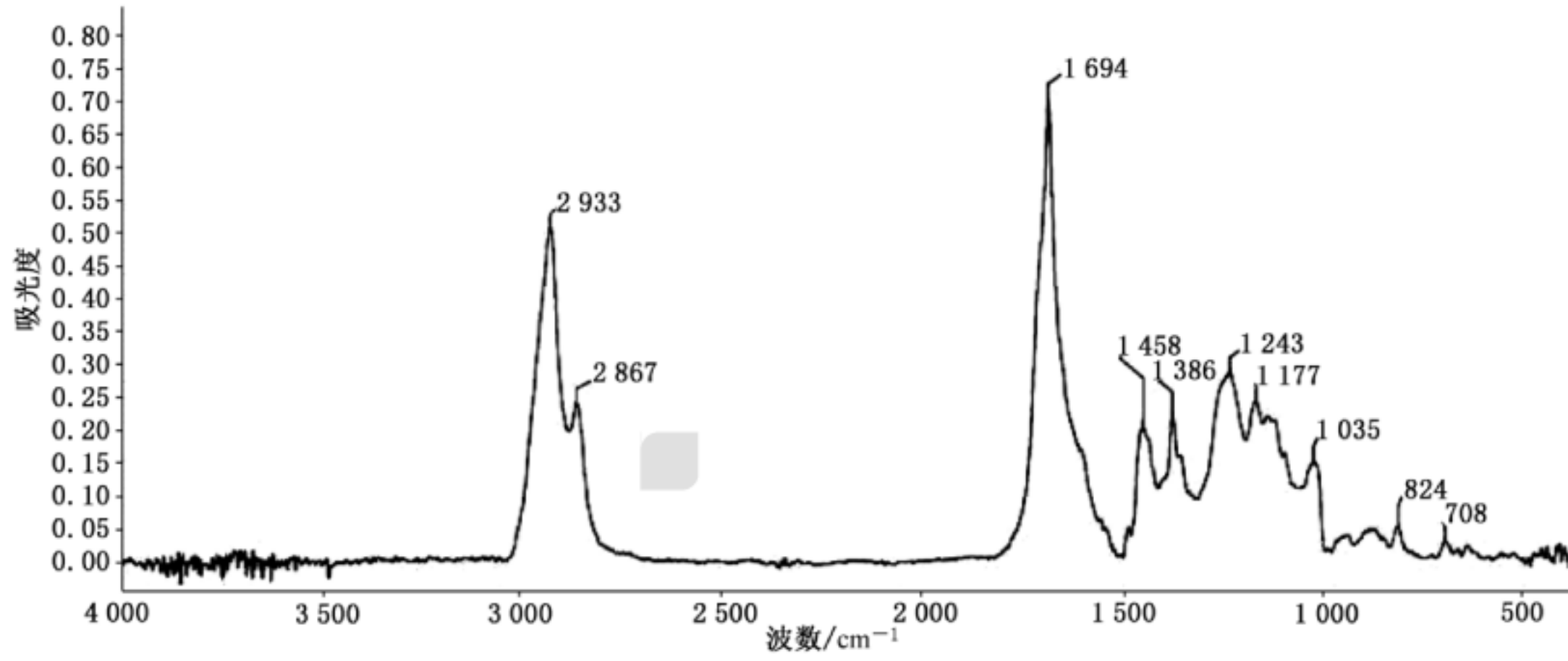
图 A.10 未石化树脂(松香)的特征红外光谱
