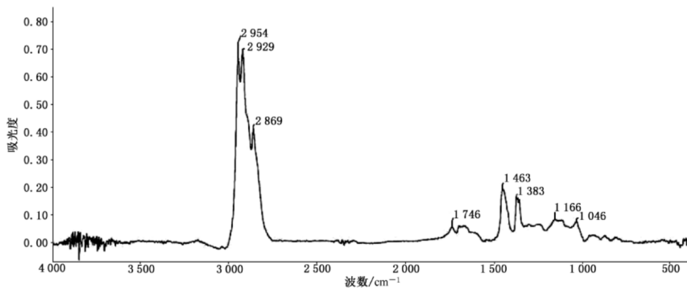
图 A.8 婆罗洲半石化树脂的特征红外光谱
