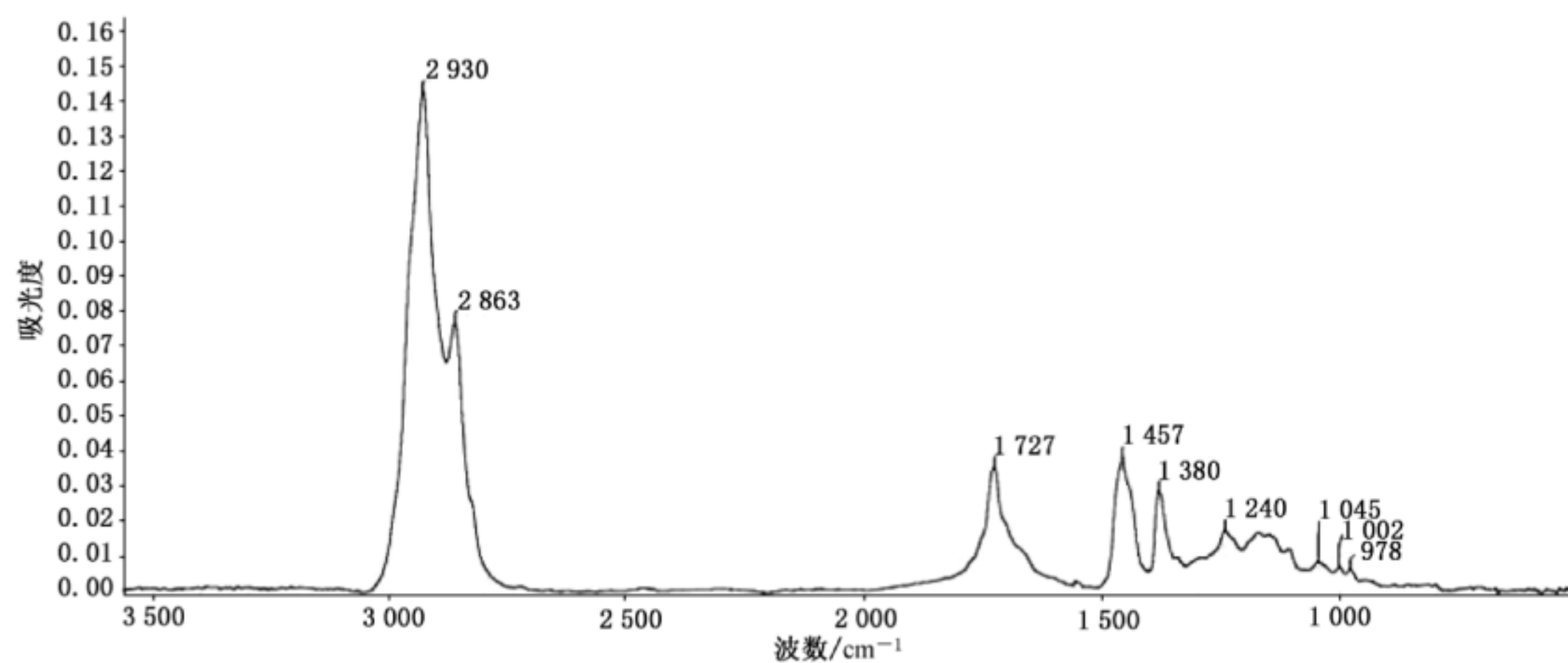
图 A.4 墨西哥目次的特征红外光谱
