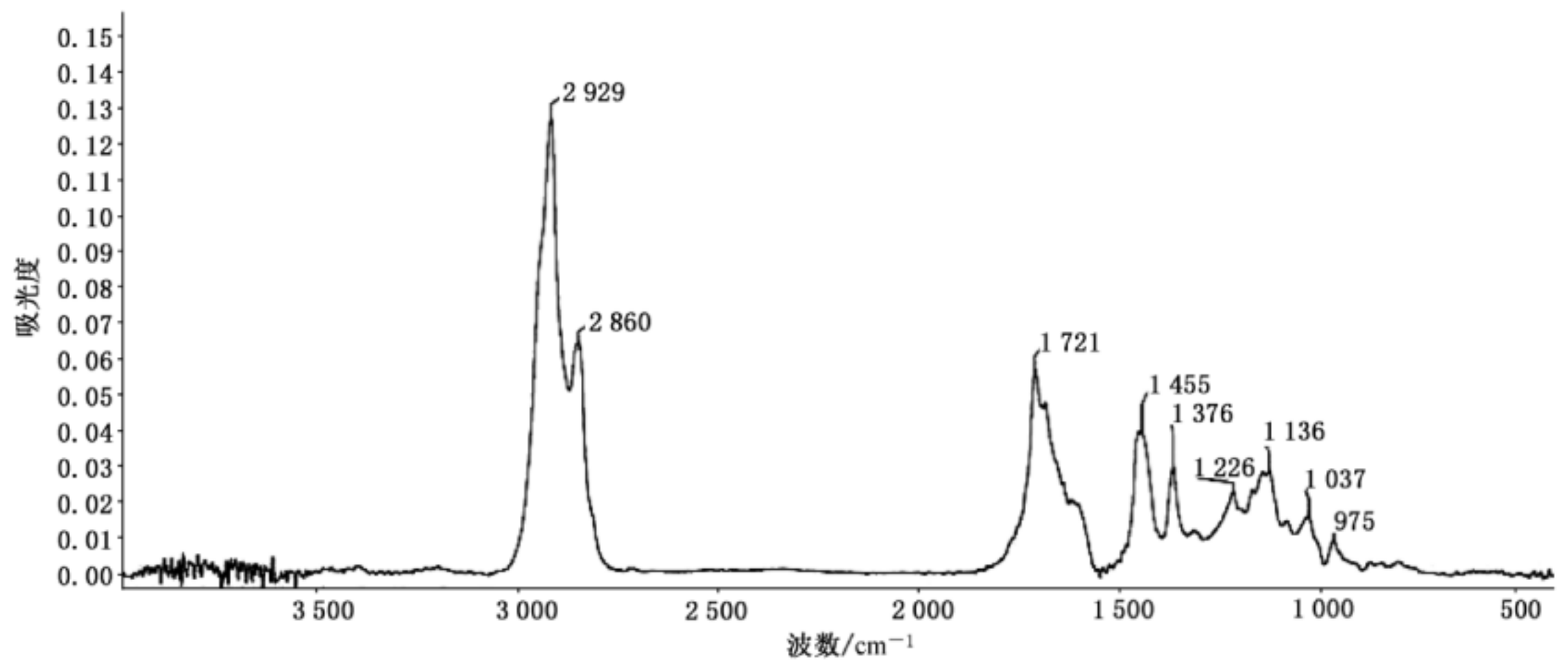
图 A.6 抚顺琥珀的特征红外光谱
