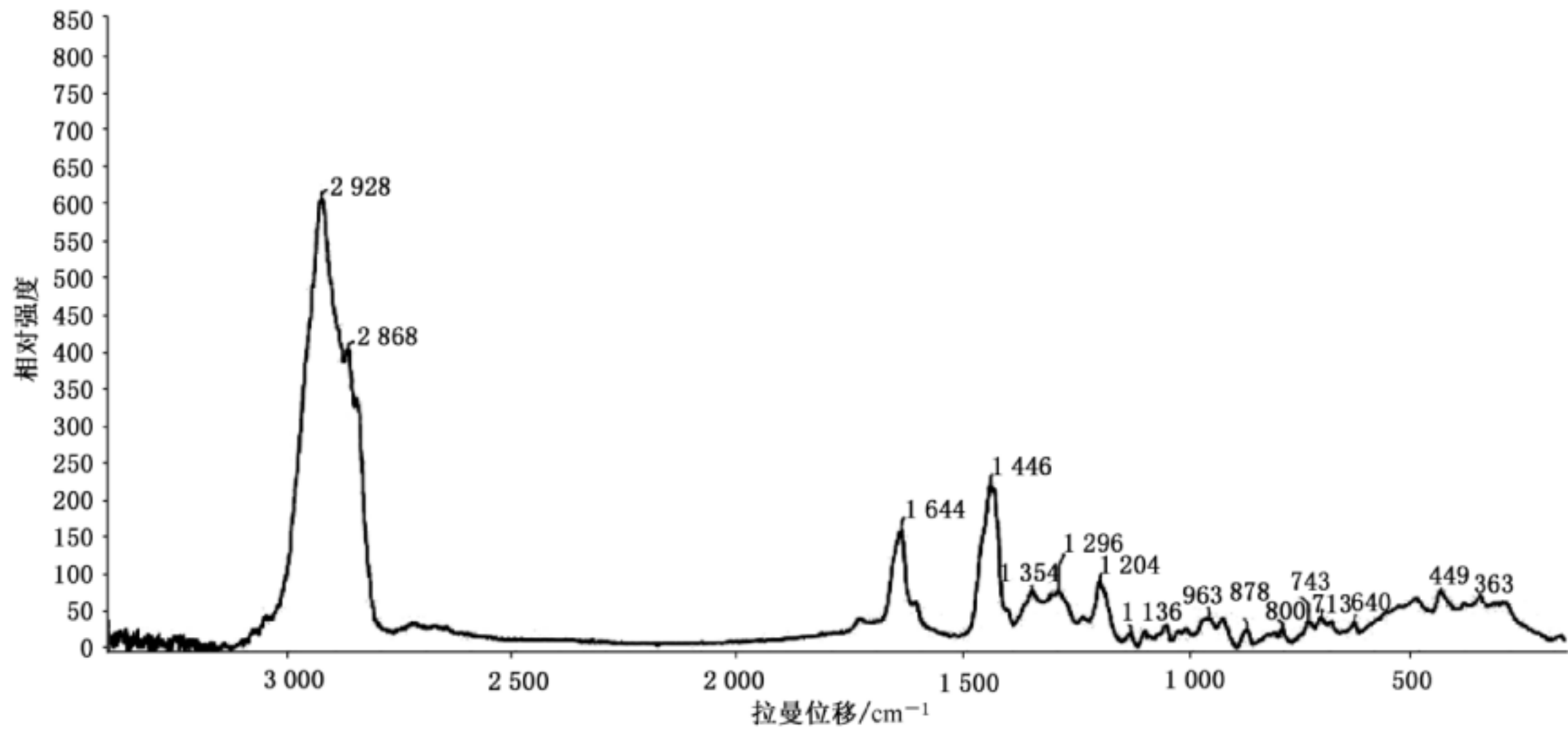
图 A.14 波罗的海琥珀(白色蜜蜡)的特征拉曼光谱
