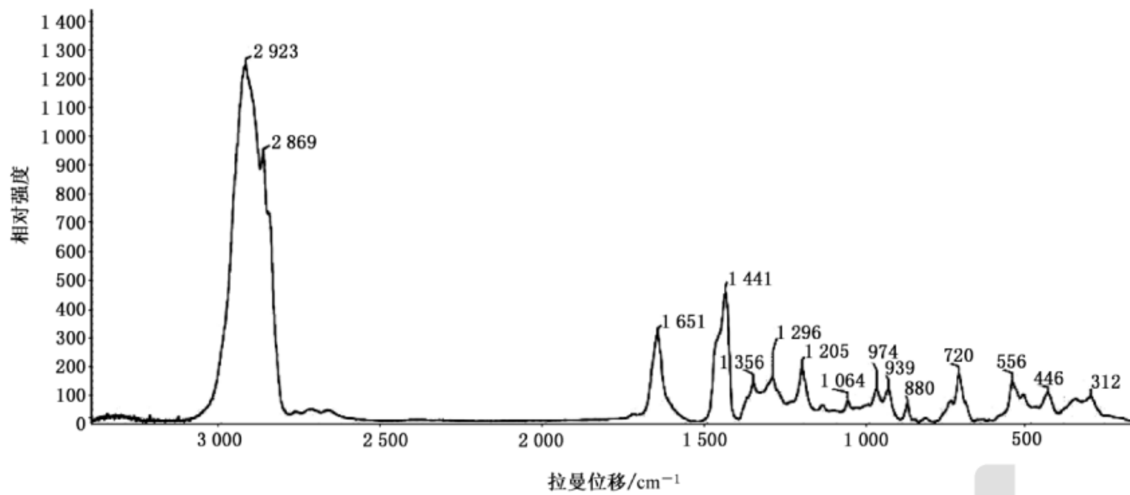
图 A.16 墨西哥琥珀的特征拉曼光谱
