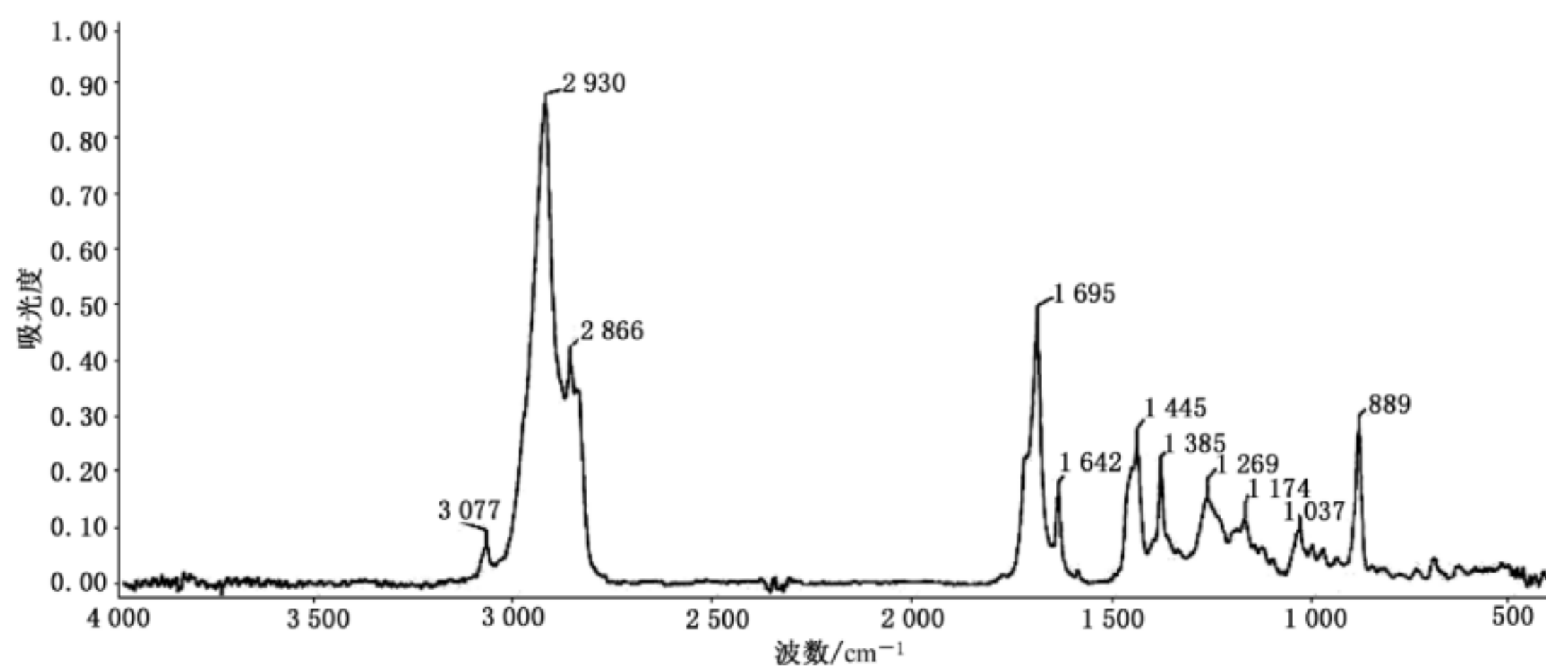
图 A.9 马达加斯加半石化树脂的特征红外光谱
