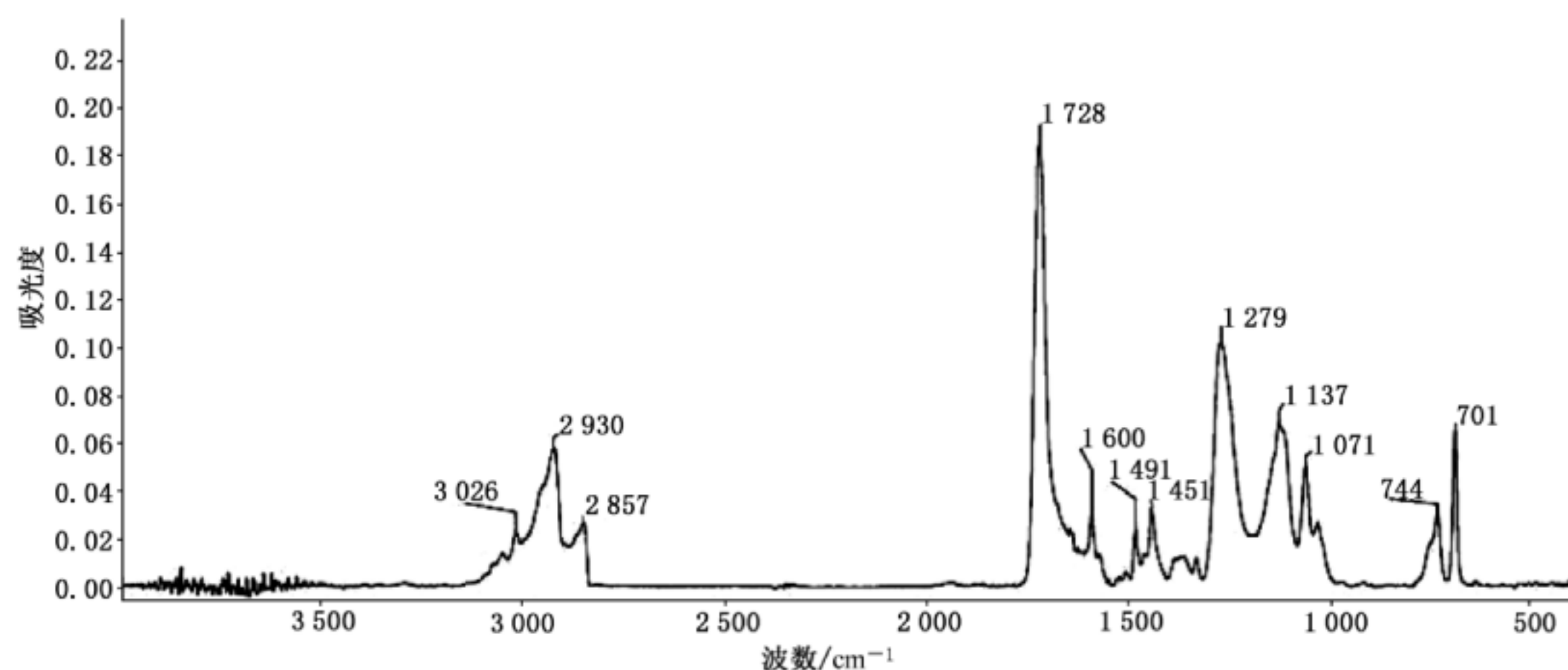
图 A.12 仿琥珀(醇酸树脂类)的特征红外光谱
