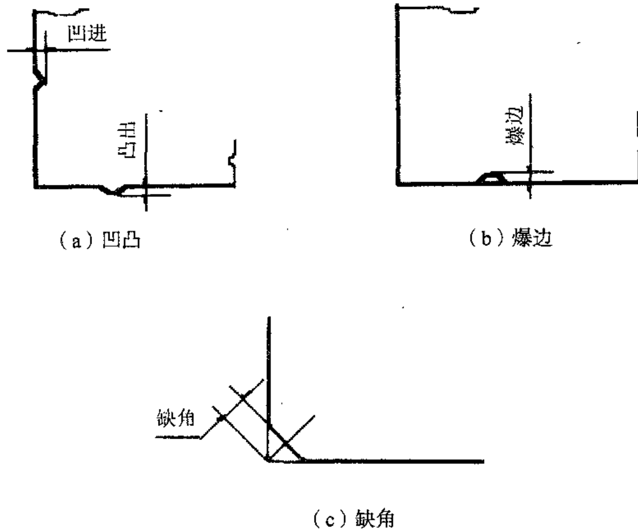
图 2 断面缺陷的测定示意图
