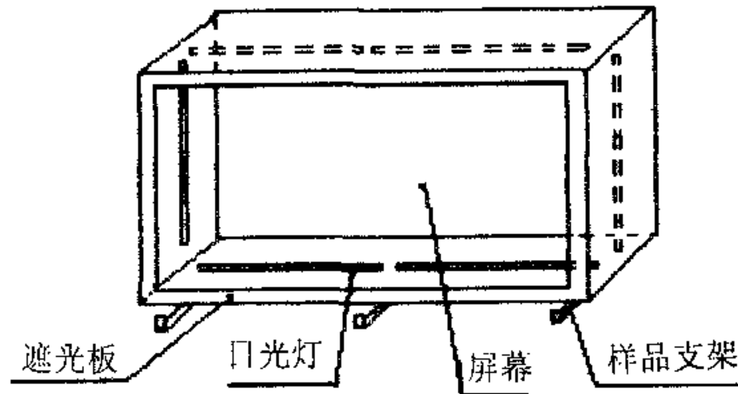
图 1 外观检验装置示意图
