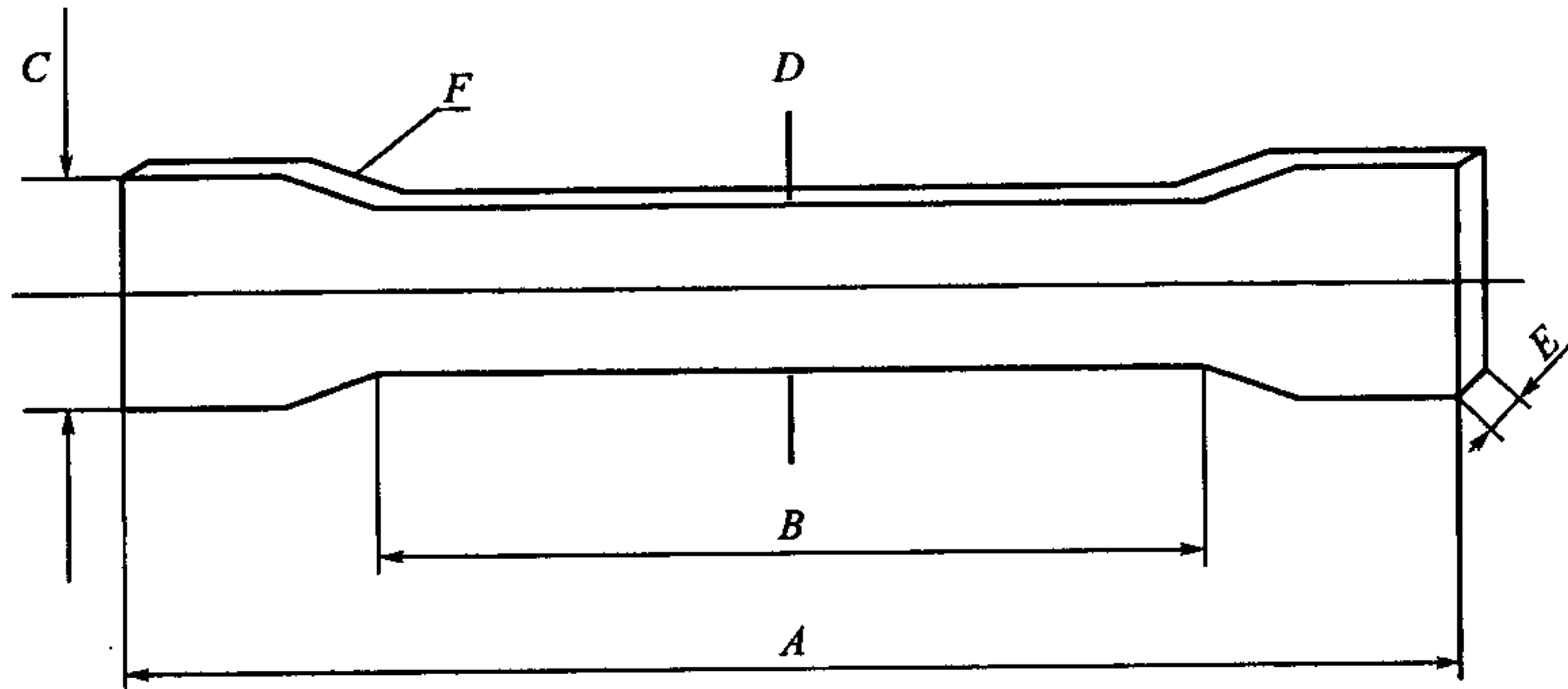
图 1 试样形状
