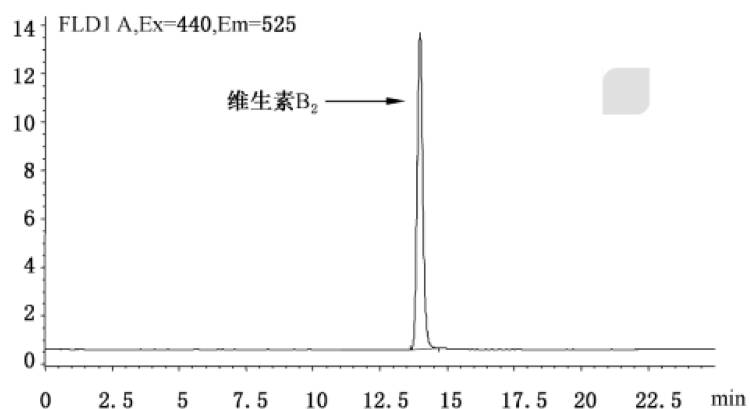
图 A.2 液相色谱荧光检测色谱条件下维生素 B 2 标准色谱图(维生素 B 2 浓度为 12 μg/mL)
