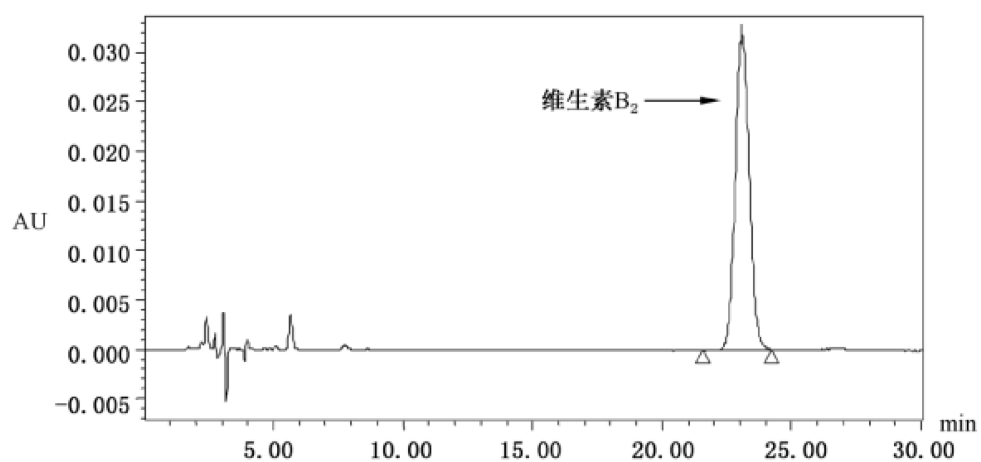
图 A.1 液相色谱紫外检测色谱条件下维生素 B 2 标准色谱图(维生素 B 2 浓度为 2 μg/mL)
