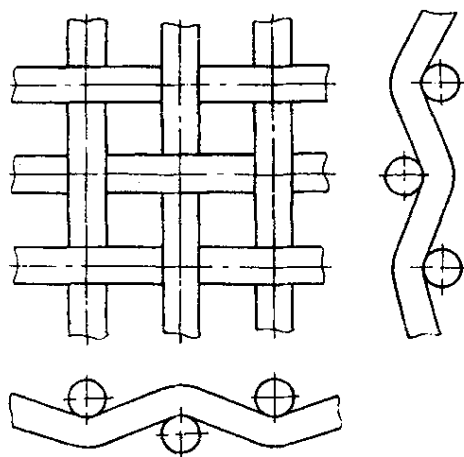
图 1 平纹编织
