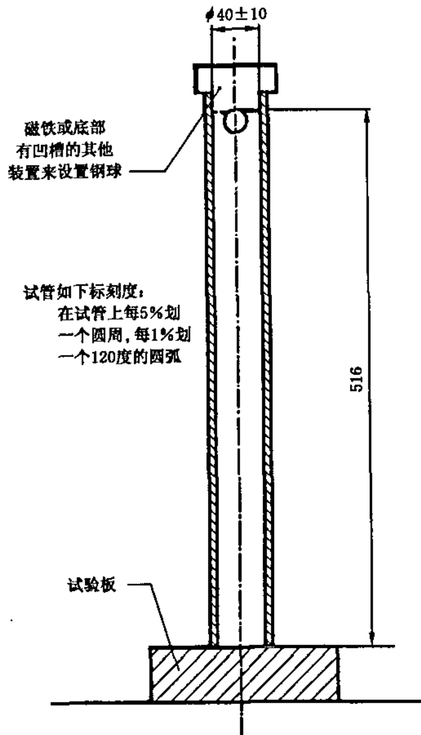
图 1 试验仪器的布置图
