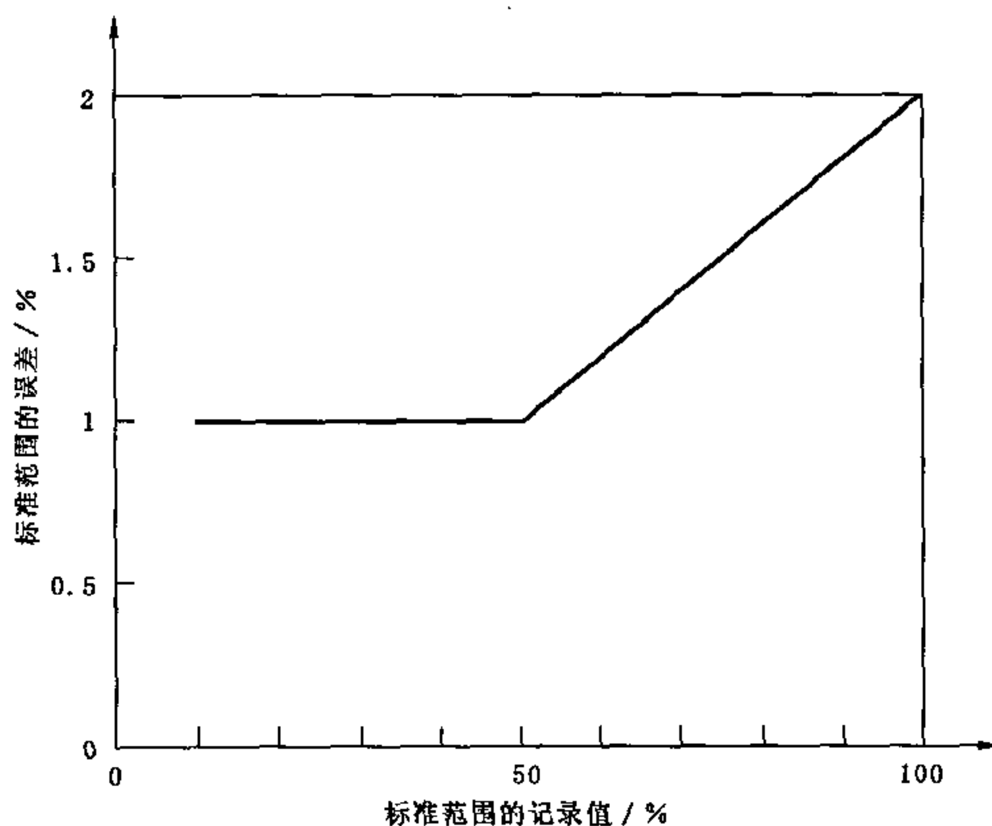
图 1 标准力范围内的记录值的允许误差
