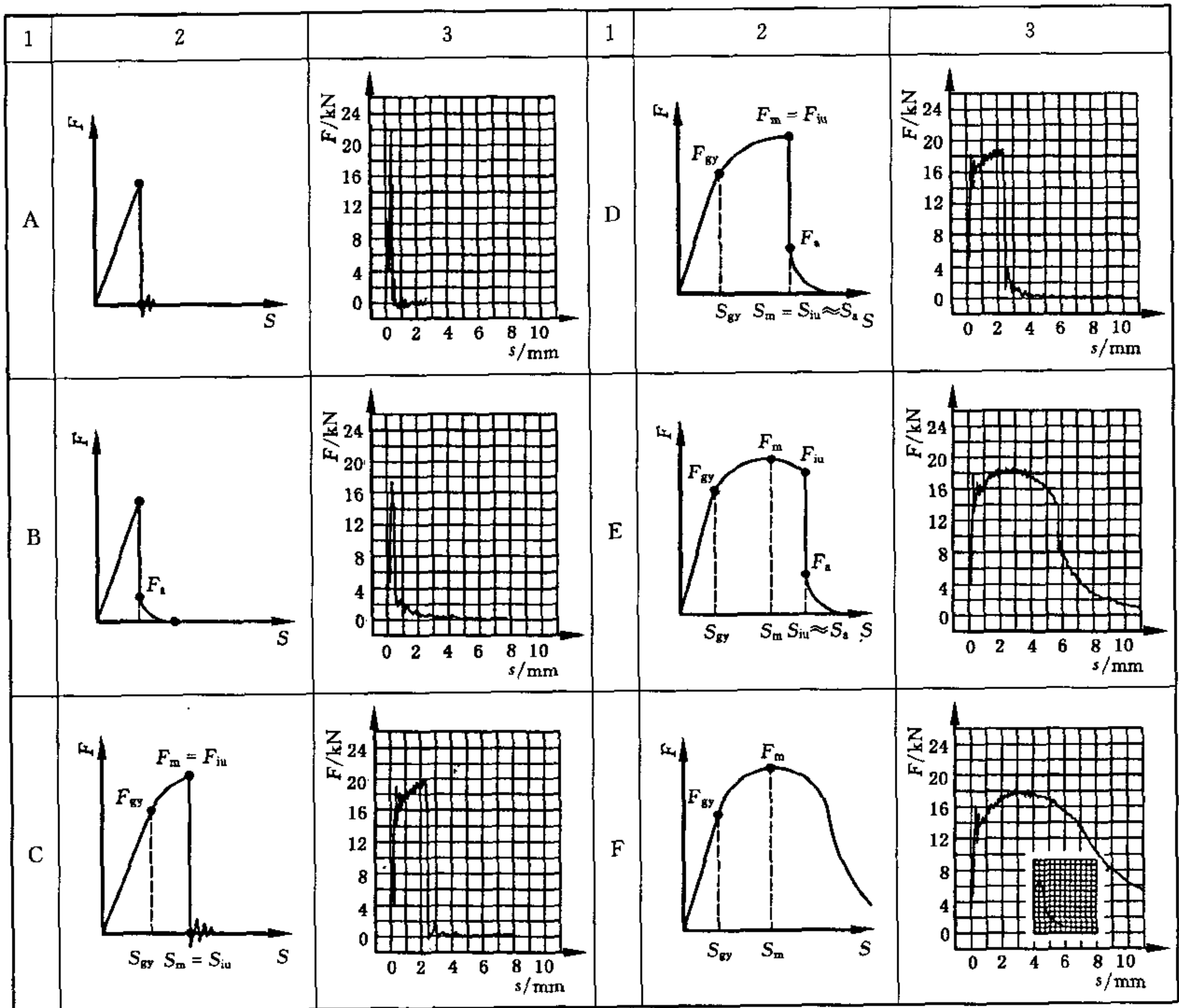
图3 力-位移特征曲线的分类
