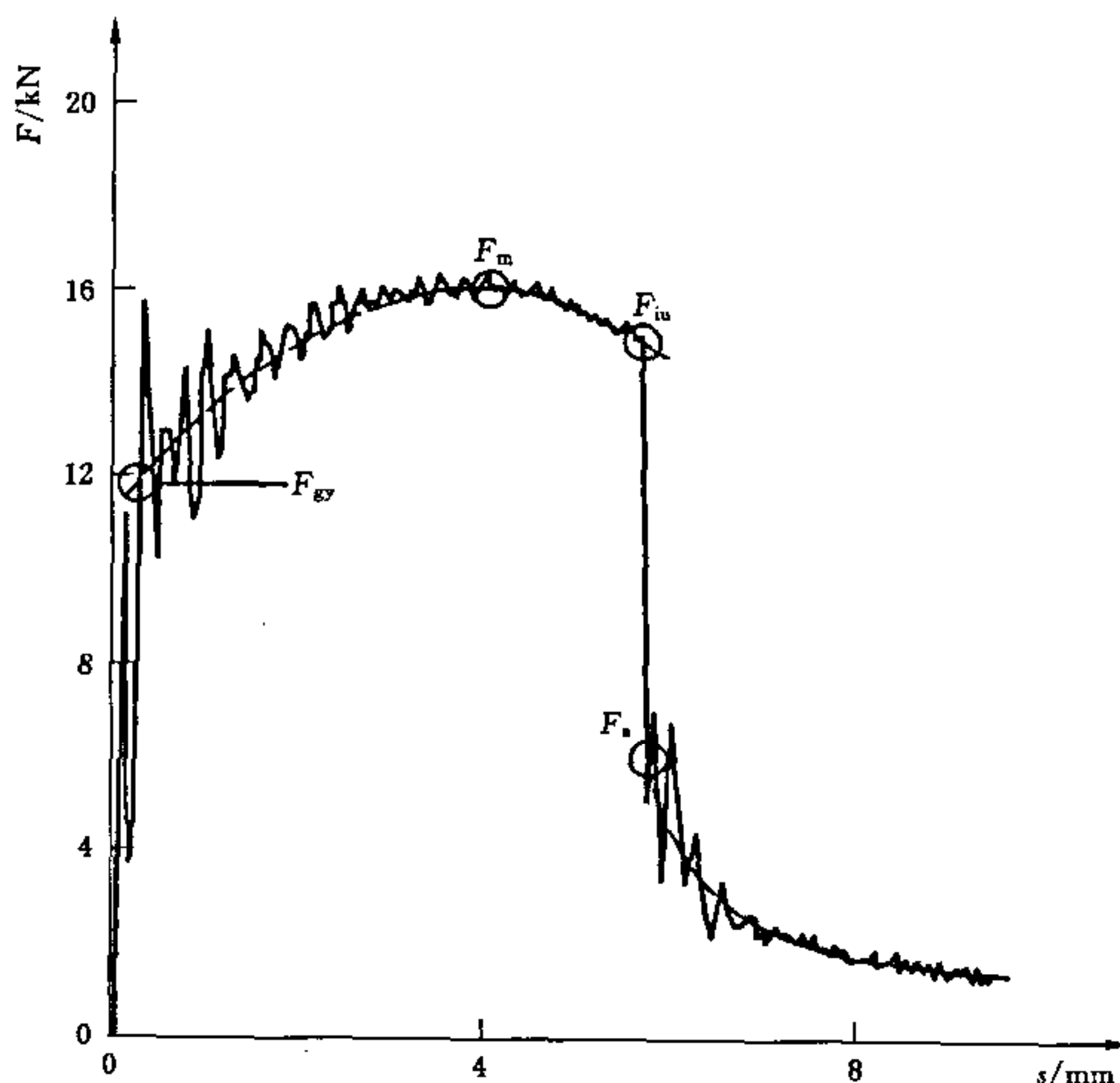
图 2 力特征值的确定
