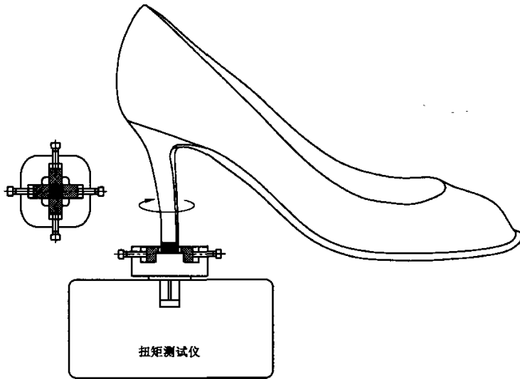
图 1 扭矩测试示意图
