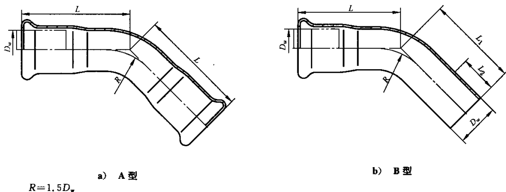
图 4 45°弯头
