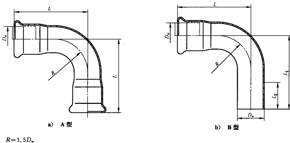
图 5 90°弯头
