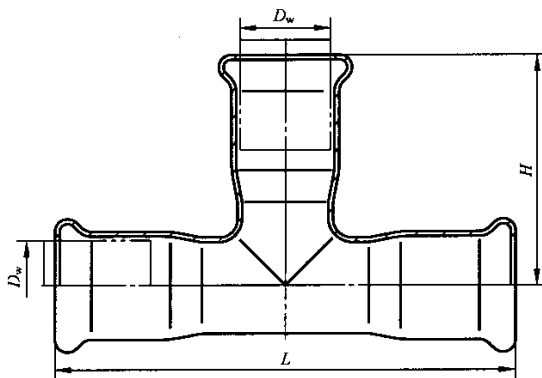
图 2 等径三通
