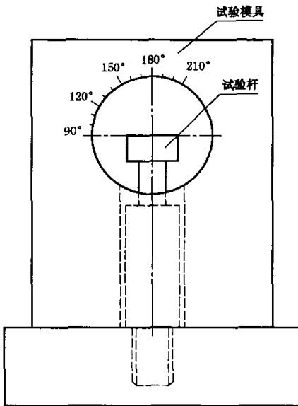
a) 未装入偏心体
