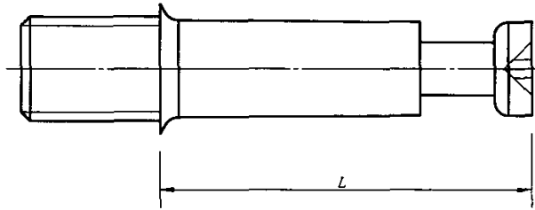
图2 无螺纹杆长度 L
