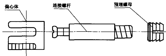
图 1 三合一偏心连接件
