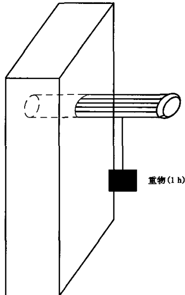
图 9 棒静载荷强度试验方法
