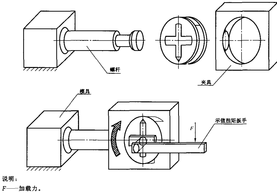
图 8 偏心体与连接螺杆的扭矩试验方法
